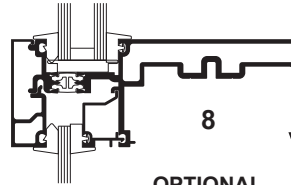
OPTIONAL HORIZONTAL
