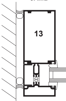
ALTERNATE JAMB
